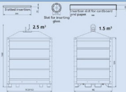
Optiune cu capac tip coa gurilor Tip 5464 – 1,5 m 3 Tip 5466 – 2,5 m 3
