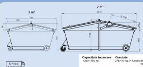
Tip 1174P cu capac plastic
